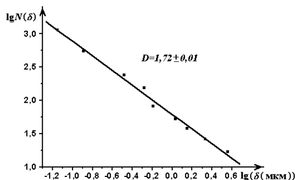
Рис. 2. Число ячеек N размером \delta \times \delta , необходимых для покрытия границ дендрита, как функция шага \delta (мкм) в логарифмических координатах
