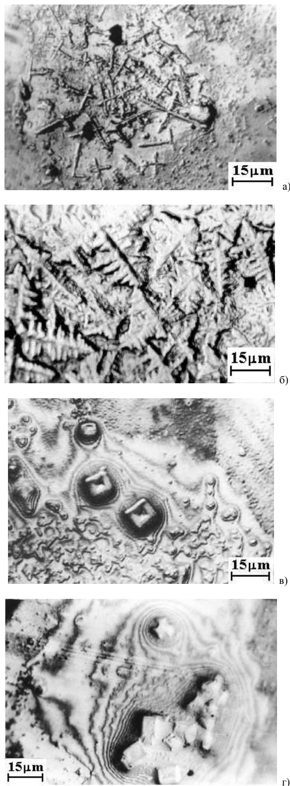
Рис. 3. Поверхность МС, содержащая локальные области с кристаллами, T_{an} = 823 К: а, б) дендриты; в, г) кристаллы правильных форм
