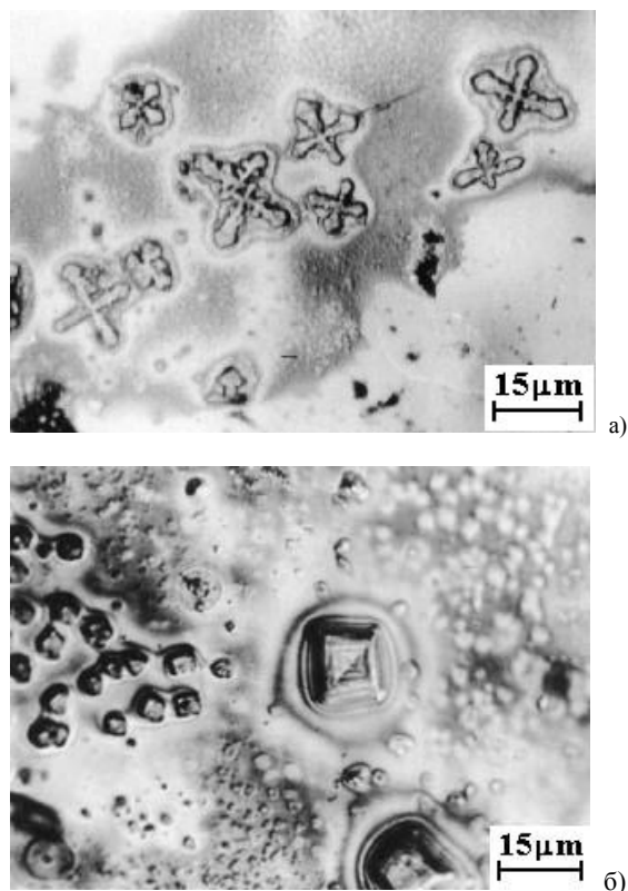
Рис. 1. Типичный вид кристаллов, выделяющихся на контактной стороне ленты МС в преддверии объемной кристаллизации
