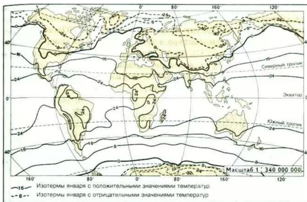
Рис. 2. Нулевая изотерма января
