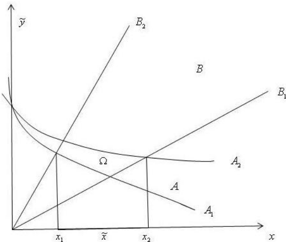
Рис. 1. Графическое представление решения интервального уравнения множественным методом: A – интервальная кривая \tilde{y} = e^{-\tilde{p} \cdot x} , где \tilde{p} = [p_1, p_2] ; B – интервальная кривая \tilde{y} = \tilde{q}x , где \tilde{q} = [q_1, q_2] ; A_1 – детерминированная кривая y = e^{-p_1 \cdot x} ; A_2 – детерминированная кривая y = e^{-p_2 \cdot x} ; B_1 – детерминированная кривая y = q_1 \cdot x ; B_2 – детерминированная кривая y = q_2 \cdot x ; \Omega – пересечение интервальных кривых A и B . x^* = [x_1, x_2] – проекция \Omega на ось X – решение интервального уравнения e^{-\tilde{p} \cdot x} = \tilde{q}x
