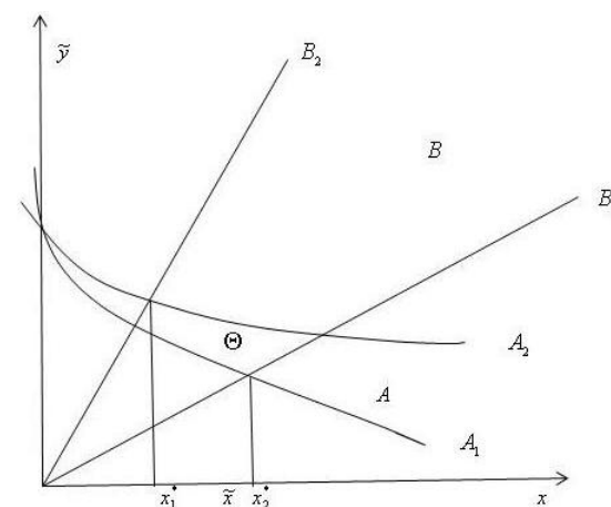
Рис. 2. Графическое представление решения интервального уравнения интервальным методом: A – интервальная кривая \tilde{y} = e^{-\tilde{p} \cdot x} , где \tilde{p} = [p_1, p_2] ; B – интервальная кривая \tilde{y} = \tilde{q}x , где \tilde{q} = [q_1, q_2] ; A_1 – детерминированная кривая y = e^{-p_1x} ; A_2 – детерминированная кривая y = e^{-p_2x} ; B_1 – детерминированная кривая y = q_1x ; B_2 – детерминированная кривая y = q_2x ; \Theta – пересечение интервальных кривых A и B . x^* = [x_1^*, x_2^*] – проекция \Theta на ось X – решение интервального уравнения e^{-\tilde{p} \cdot x} = \tilde{q}x
