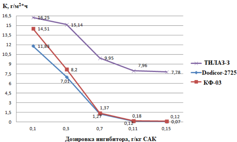
Рис. 1. Зависимость скорости коррозии стали СтЗпс от дозировки ингибиторов в среде 10 %-ной сульфаминовой кислоты
